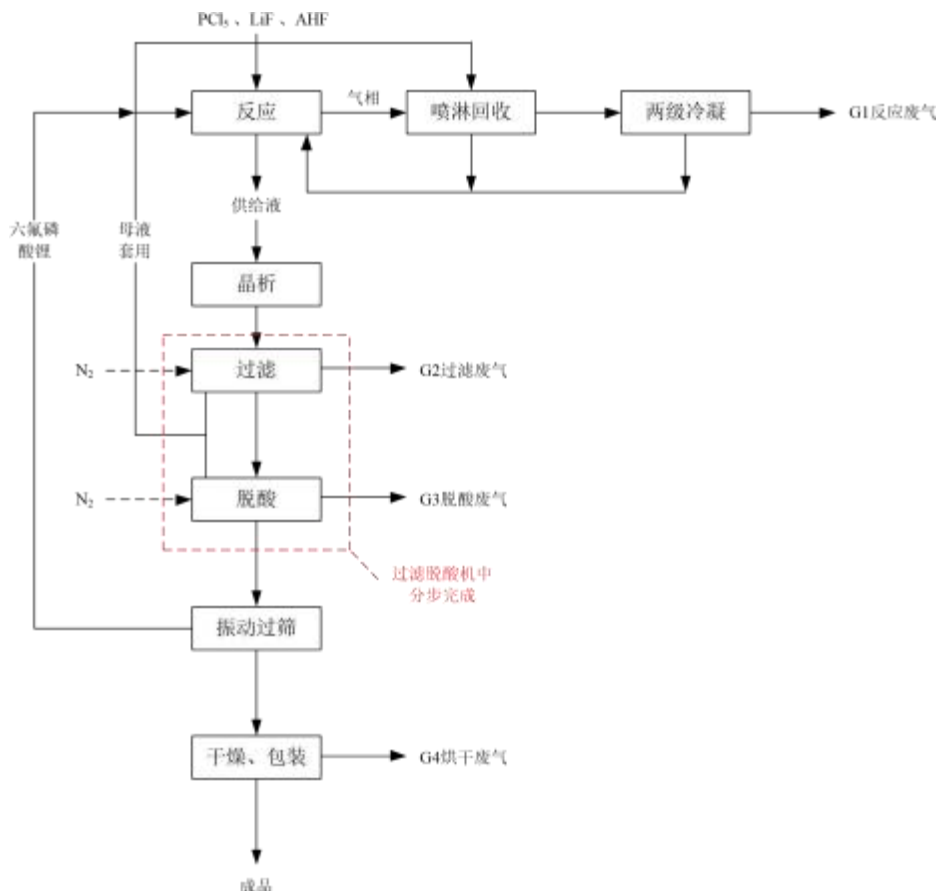
图 4.1-1 生产工艺流程图
