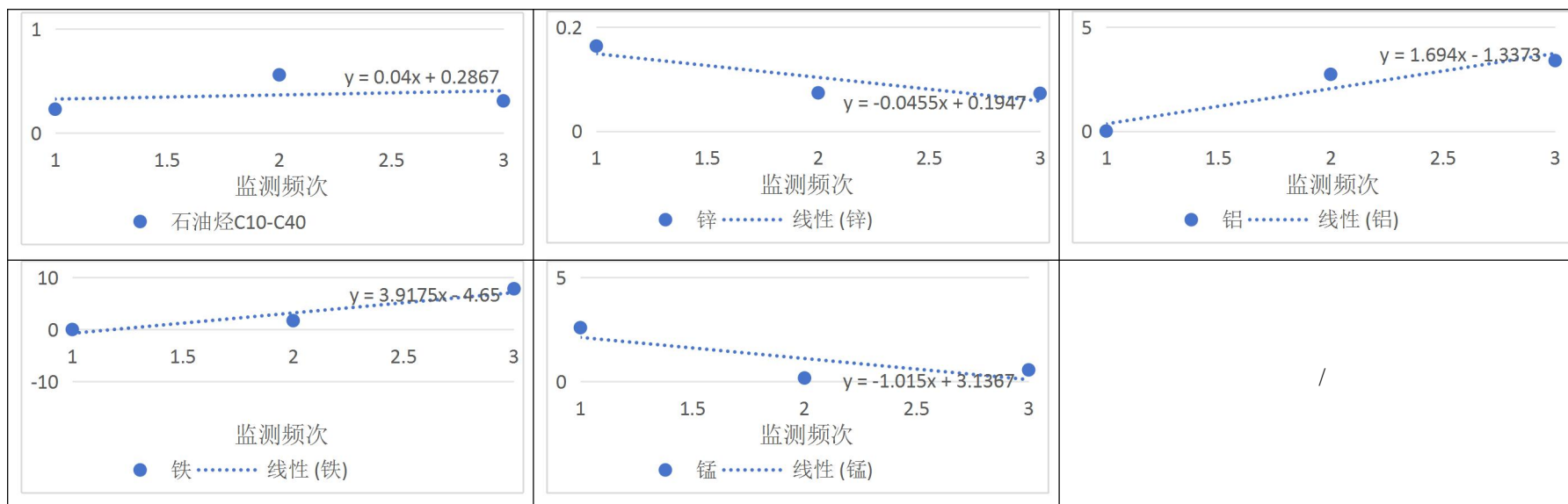
图10.2-3 地下水GW3点位污染物浓度监测值变化及趋势预测图
