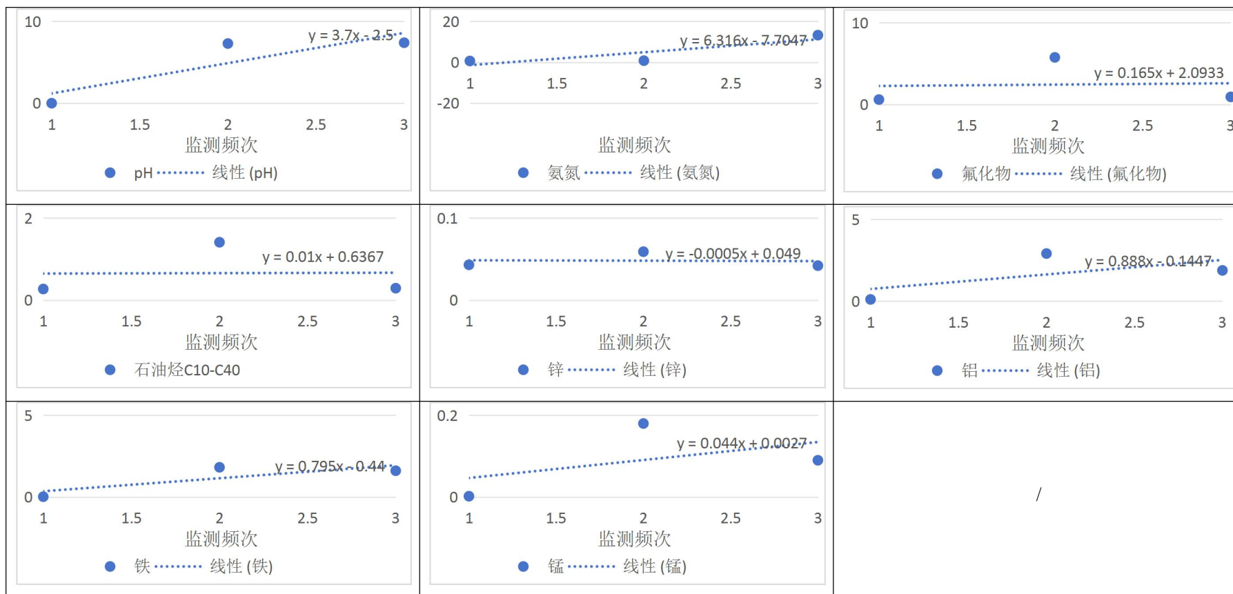
图10.2-1 地下水GW1点位污染物浓度监测值变化及趋势预测图
