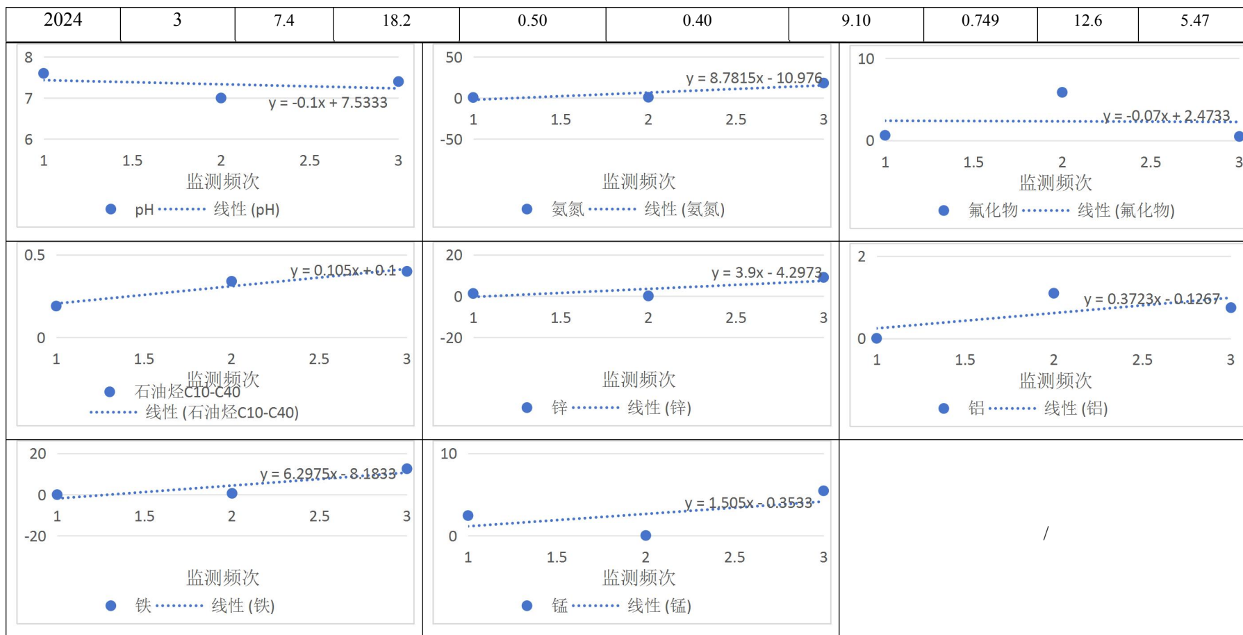
图10.2-4 地下水BGW1点位污染物浓度监测值变化及趋势预测图
